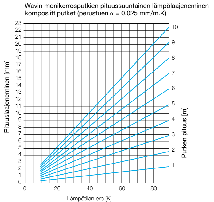
Kuva 36: Pituussuuntainen lämpölaajeneminen.
