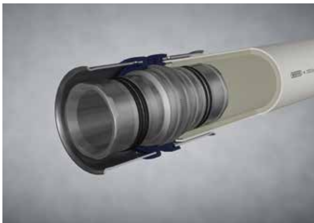
Kuva 17: Alhainen sisäänvientivoima patentoidun kuusikulmisen holkin pään ansiosta.
