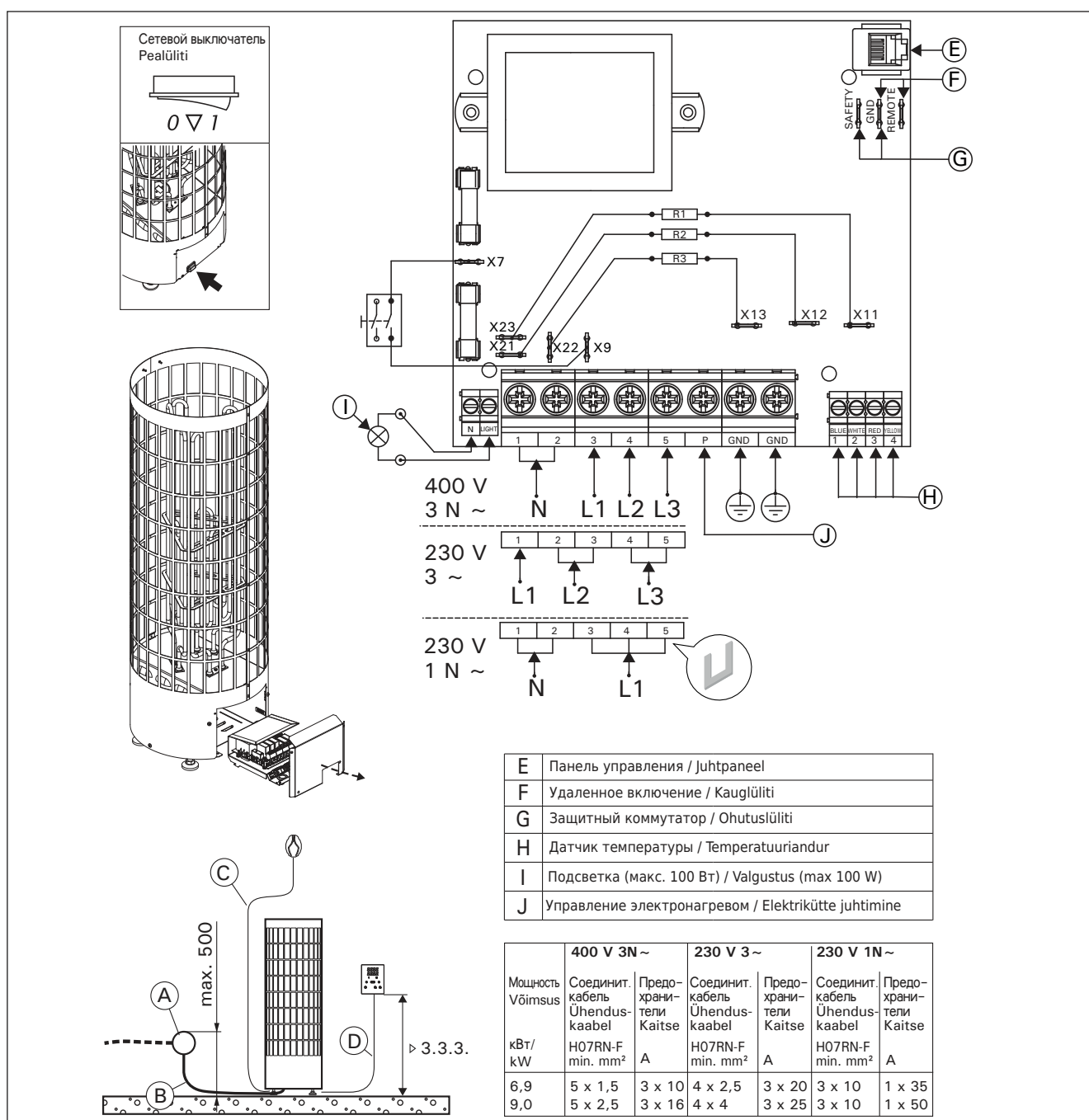
Рисунок 7. Электромонтаж Joonis 7. Elektriihendused
