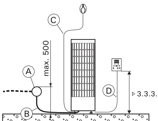
Kuva 7. Sähkökytkennät Bild 7. Elinstallationer
