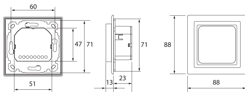
Danfoss Icon™ Display 088U1012 (sis. Feller EDIZIOdue -kehyksen ja -sovittimen)
