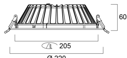
Ø 220 Insaver Slim 205 pyöreä
