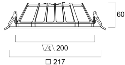
□ 217 Insaver Slim 200 neliö
