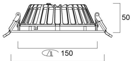
Ø 164 Insaver Slim 150 pyöreä
