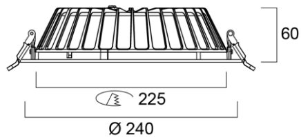
Ø 240 Insaver Slim 225 pyöreä
