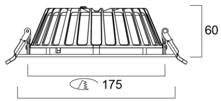
Ø 193 Insaver Slim 175 pyöreä
