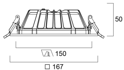
□ 167 Insaver Slim 150 neliö
