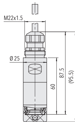
OEM-version
