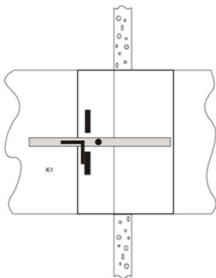
Palopelti auki K1: 13/14 kiinni 21/22 auki
