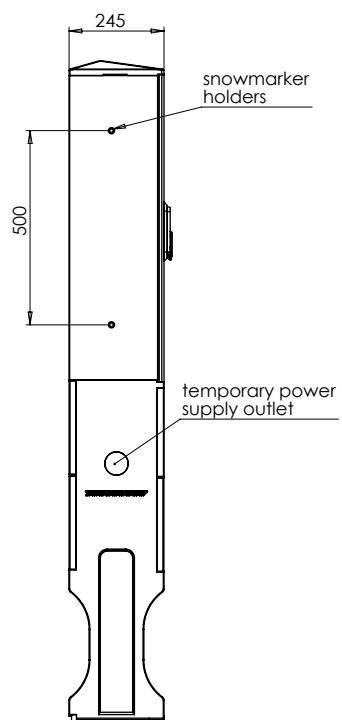
OKKJK-P 250A 26x80 BC+160
