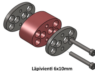
Läpivienti 6x10mm
