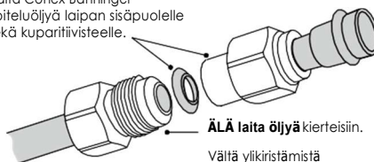
Kuva 2. Ruostumaton teräslaippa ja kuparitiiviste.
