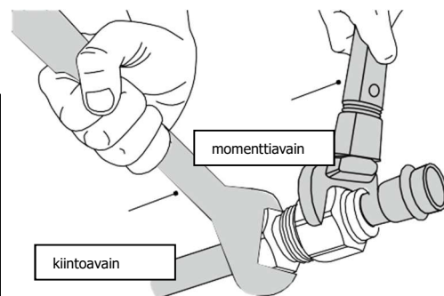
Kuva 3. Kiristä liitos momenttiavaimella.
