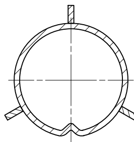
A-A (1:2)
