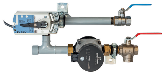
Lämmityksen säätöryhmä Aries, Qi ja LSR Si KV4
