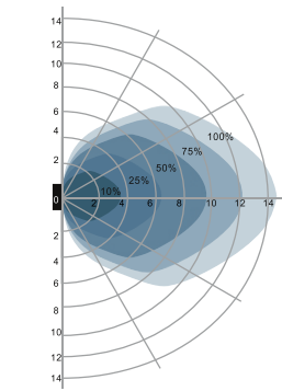
Detektionsmönster vid takmontering (enhet: m) Förslag till installationshöjd: 1–1,8 m
