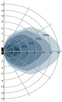
Krzywa dla naściennego sposobu instalacji. Sugerowana wysokość montażu: 1–1,8 m
